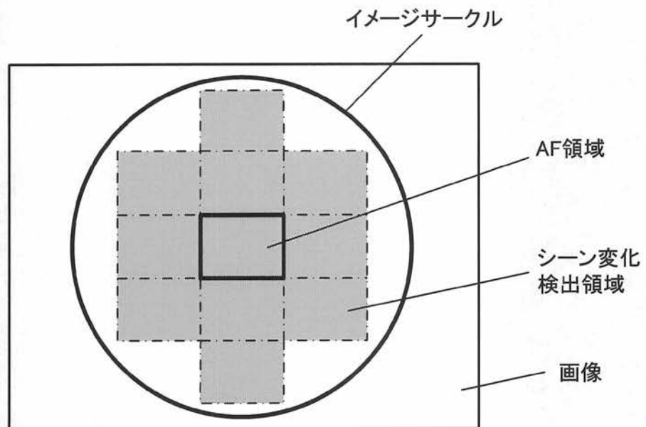
イメージサークル径が小さい場合
